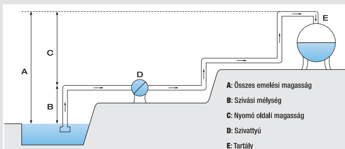
Az átemelő szivattyúk elvi működése
